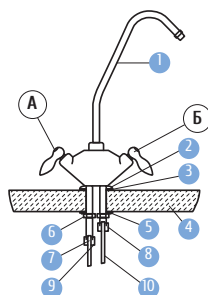
ДВУЛУЧЕВОЙ КРАН
